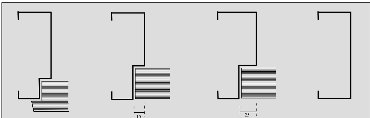
Standaard opdek
