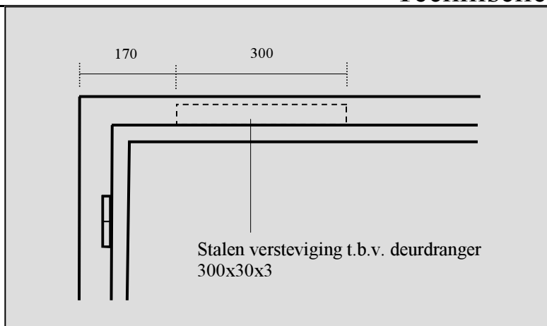
Deurdranger voorziening
