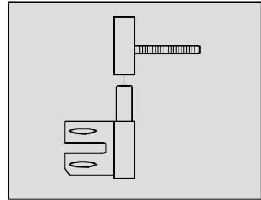
Paumelle t.b.v. opdek inmetselekozijnen. Paumellekastje is aangelast.
