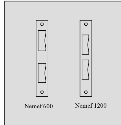
Type schootplaat bij stompe kozijn
